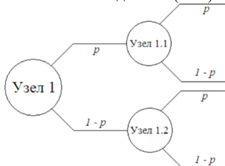
Рисунок - Дерево вероятностей
