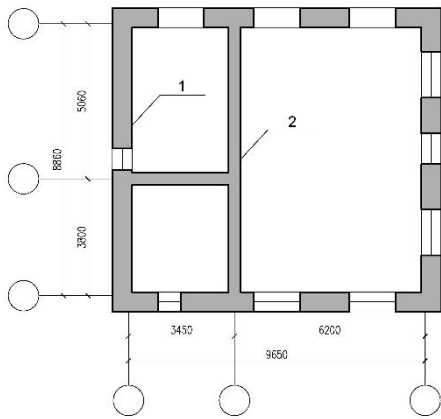
План 1 этажа
