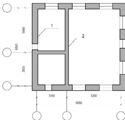
План 1 этажа
