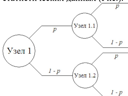
Рисунок - Дерево вероятностей
