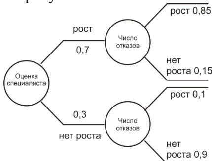
Рисунок 4.2 - Бинарное дерево вероятностей
