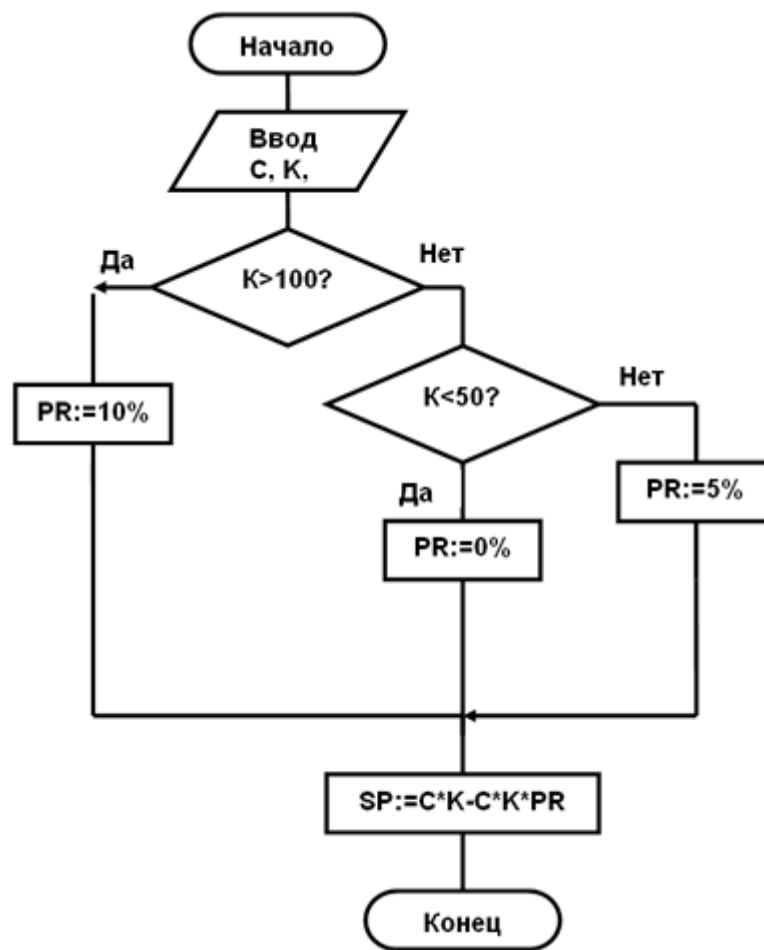
Рис. 3. Вложенные условия
