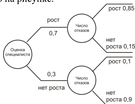
Рисунок 4.2 - Бинарное дерево вероятностей
